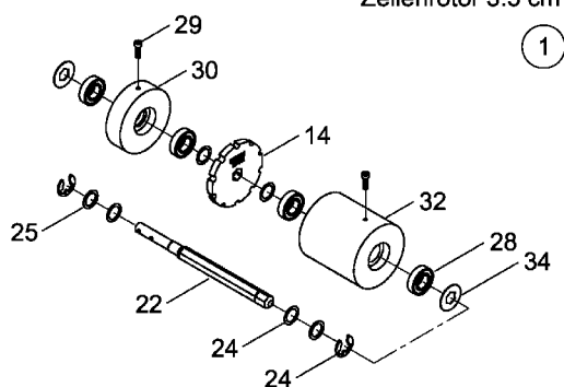
Zellenrotor 3.5 cm 3
