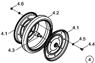
Druckrolle 2 x 13" (5cm)
