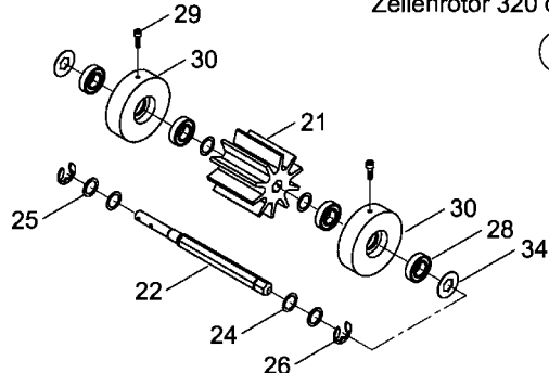
Zellenrotor 320 cm 3
