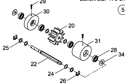
Zellenrotor 170 cm 3
