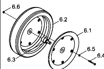
Druckrolle 3 x 13" (7,5 cm)
