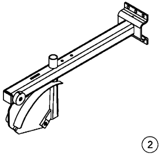
Scharkörper lang
